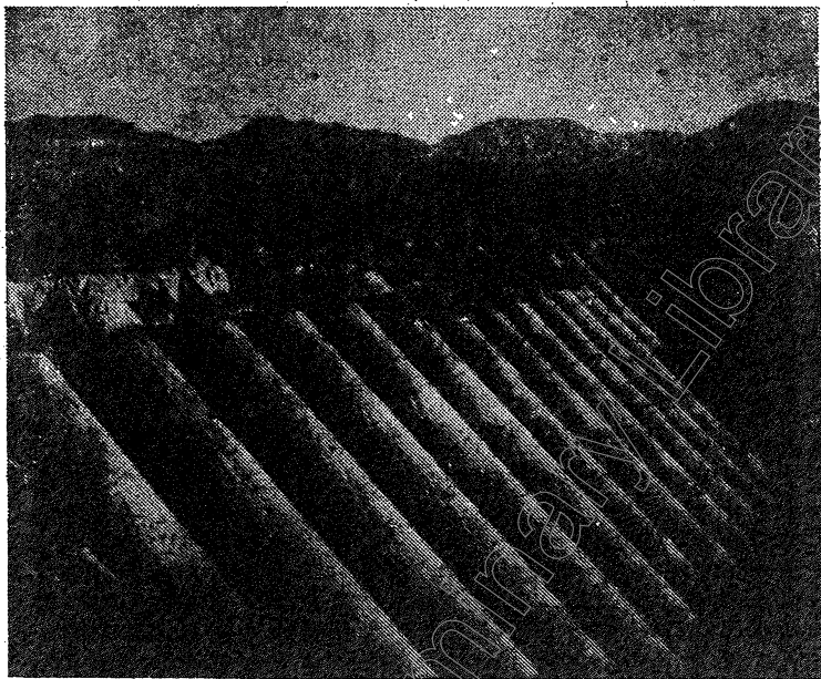
梅山水庫連拱壩近貌
